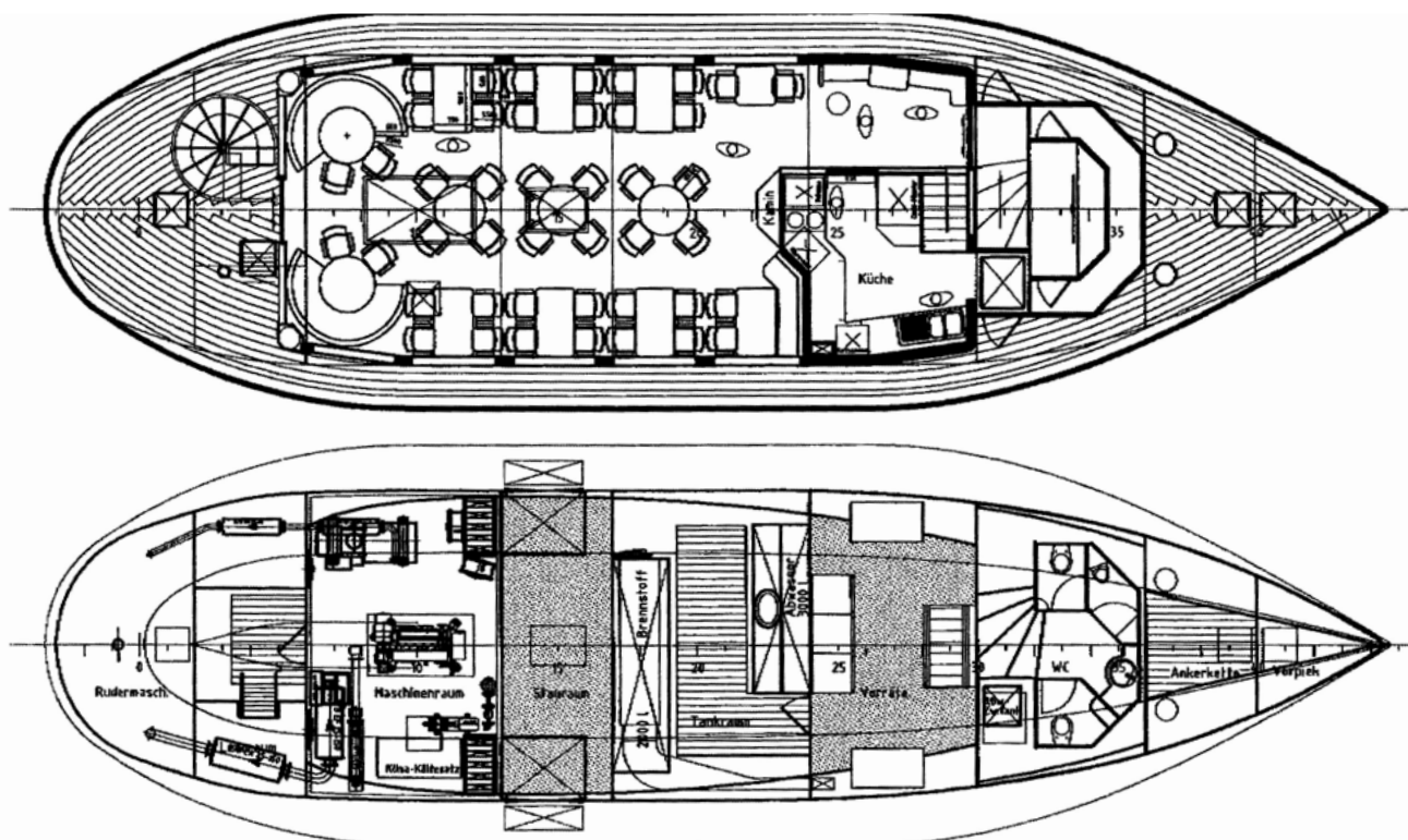
Grundriss der M.Y. «Emily»
